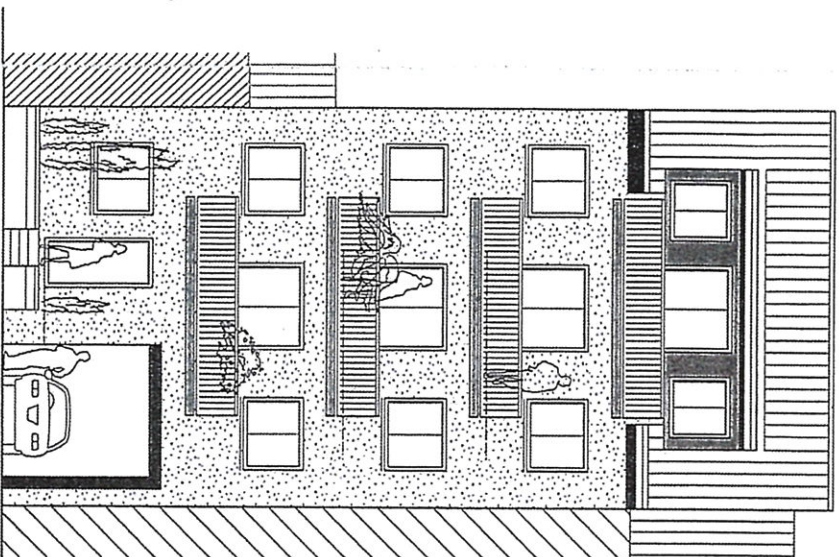
ANSICHT HOF-SEITE M. 1/ 100
