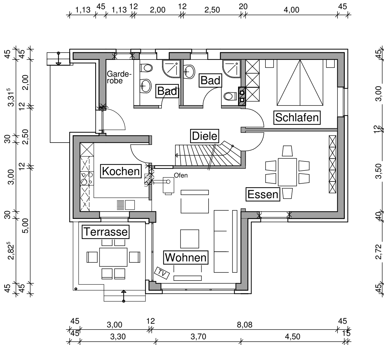
Erdgeschoss
