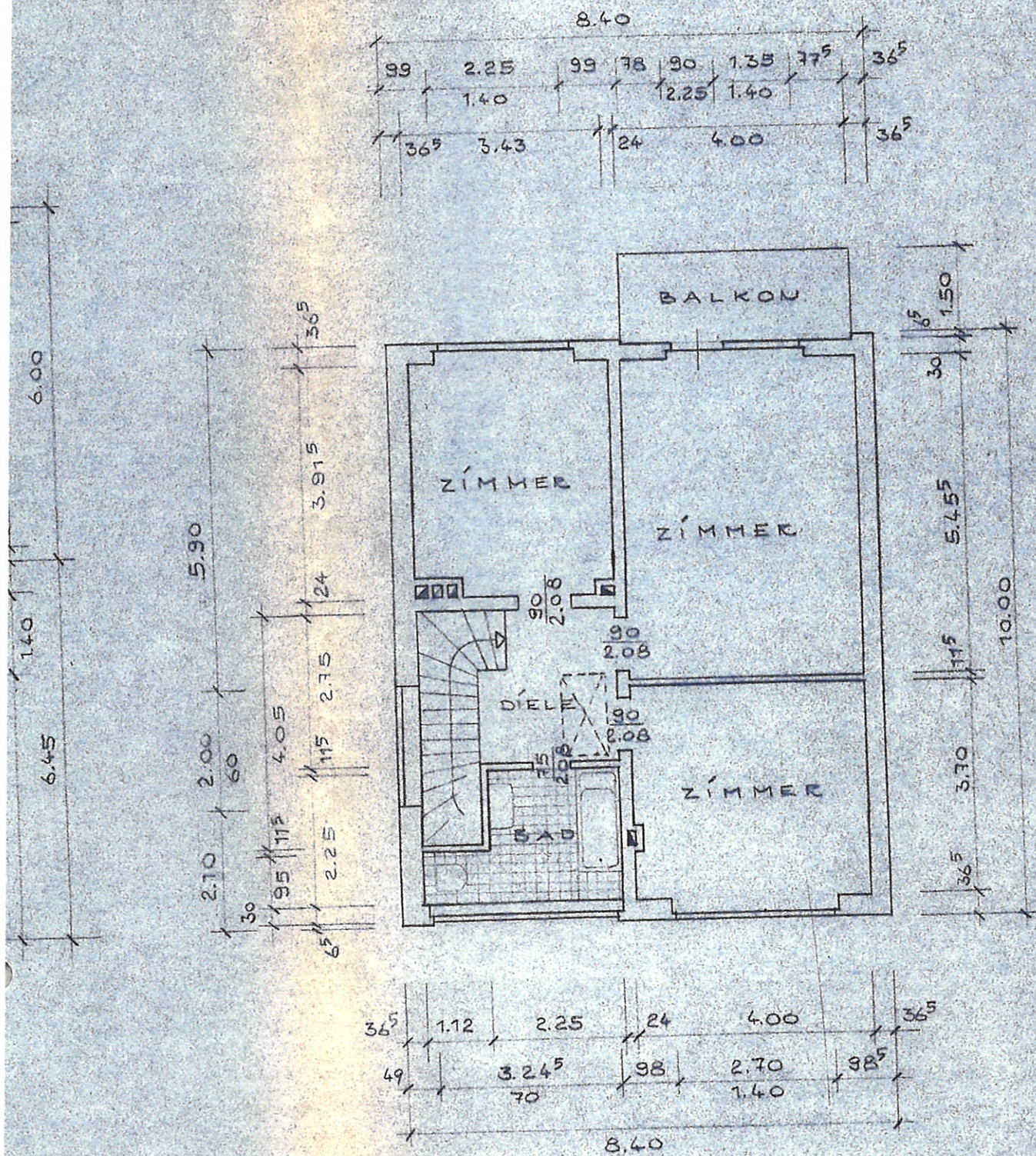
1. OBERGESCHOSS
