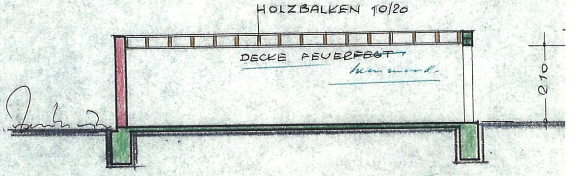
SCHNITT A-A
