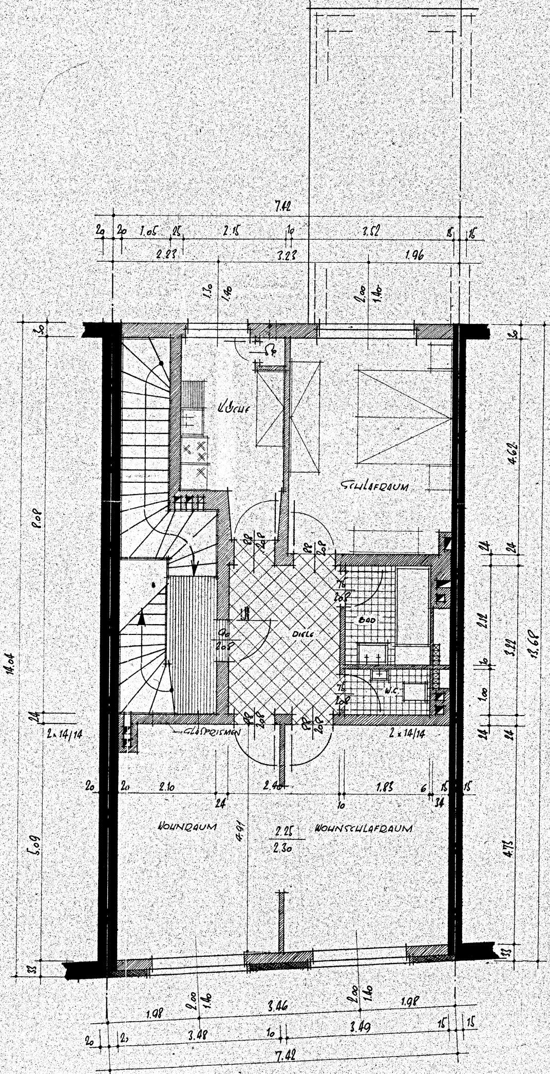
1. OBDRGESCHOSS
