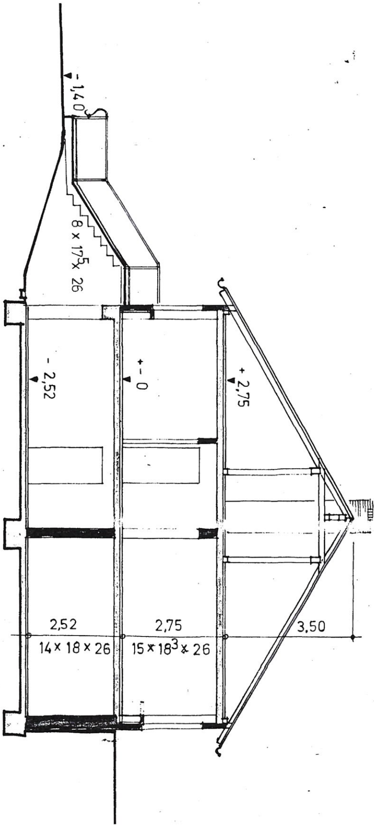
SCHNITT "A-B"
